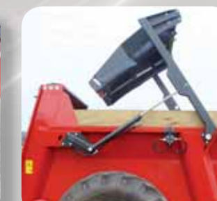
Porte hydraulique articulée
